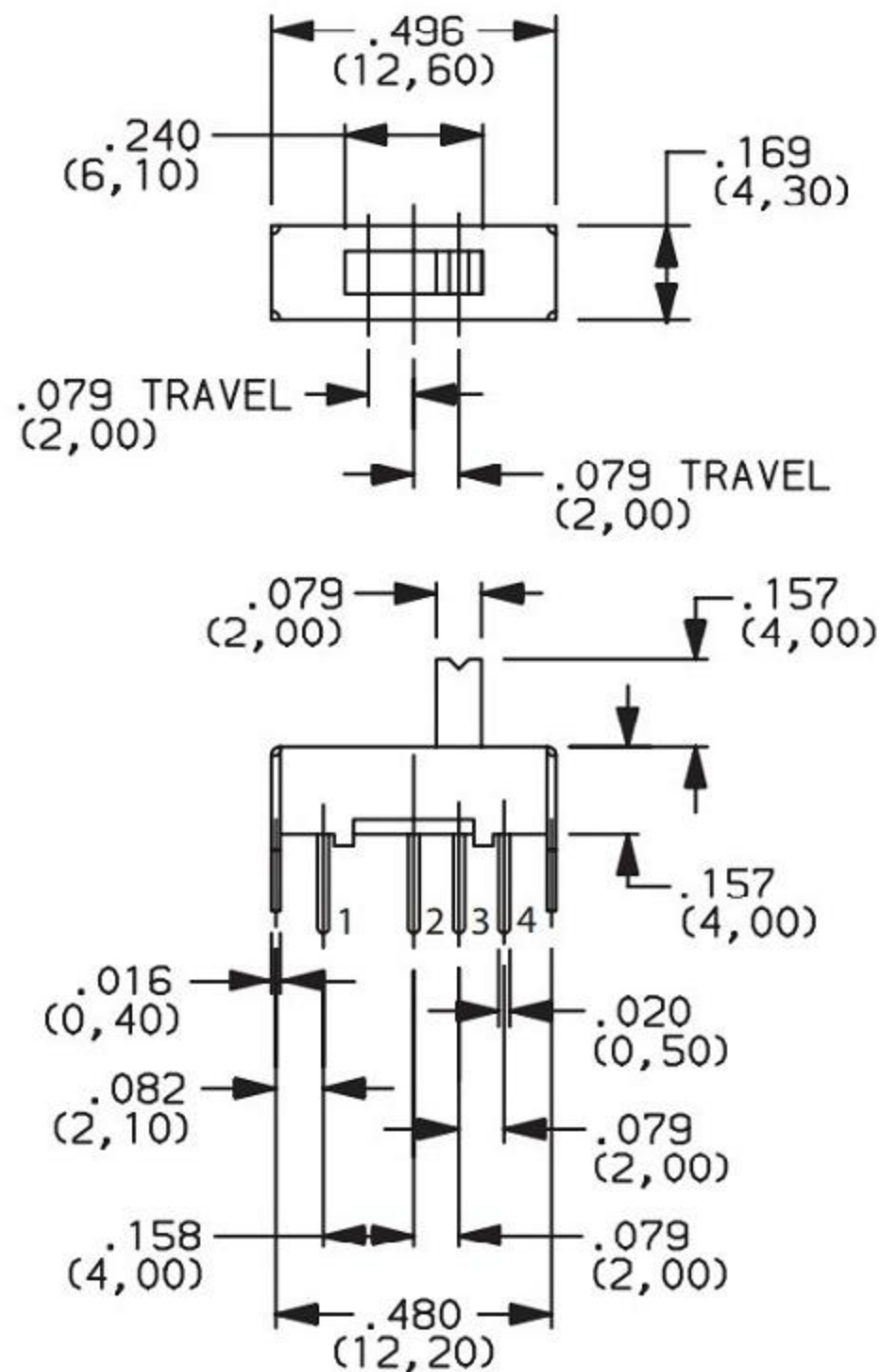
Actuator shown in pos. 3
